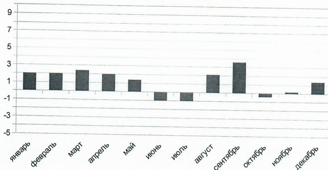
Рис. 2. Аномалии среднемесячной температуры воздуха ( ^{\circ}\text{C} ) за 2023 год
